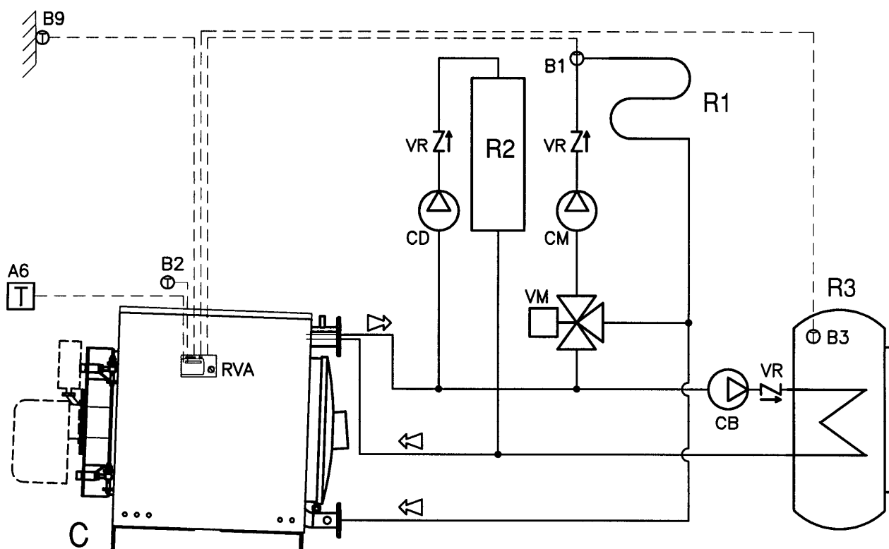
Fig. 7 - Schema d'impianto
